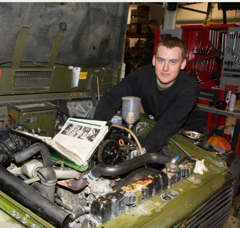
David Anker forsøker å time en dieselpumpe.
